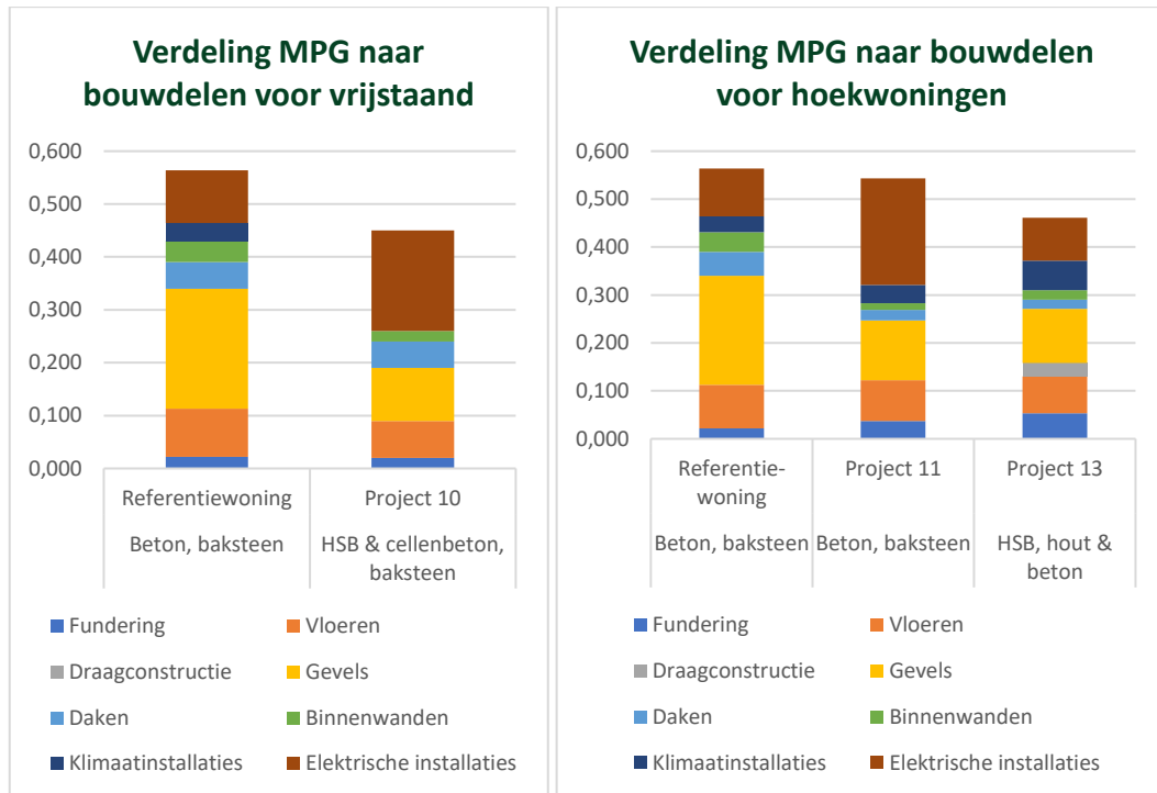
Figuur 2-8 en figuur 2-9: Verdeling MPG naar bouwdelen voor vrijstaande woningen en hoekwoningen
